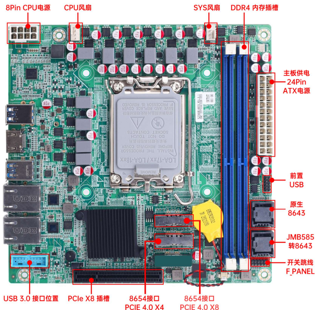
侧面接口定义分布图
