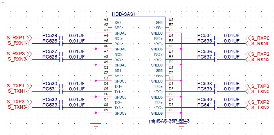
1. HDD-SAS2 8643 座子定义 (接四个 SATA HDD)
